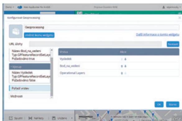
Obr. 2. Při začlenění geoprocessingu je možné ovlivnit pořadí vykreslování vstupních a výstupních vrstev.
